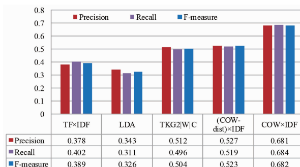
图2 英文数据集上不同算法性能对比
